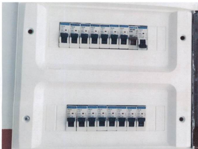
Foto 31: Disjuntor monopolar tipo DIN, corrente nominal de 16 A e de 25 A. (Itens 10.9 e 10.11)
