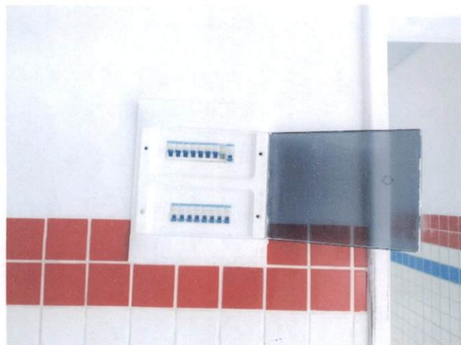
Foto 35: Quadro de distribuição de energia em PVC, de embutir, para 24 disjuntores DIN; incluindo disjuntor monopolar tipo DIN, corrente nominal de 50 A. (Itens 12.2.1 e 12.2.2)
